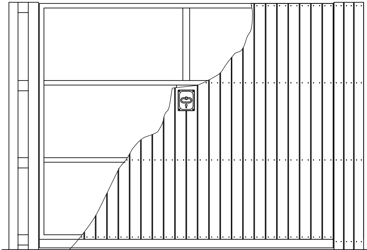
Glattkantverbreterung (Ausf. "IL" bzw. "IF")
