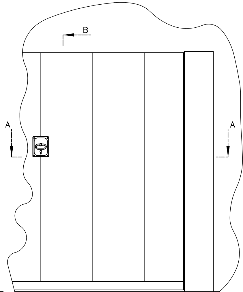
Prallschutzpaneele 470mm breit (Ausf. "DF")
