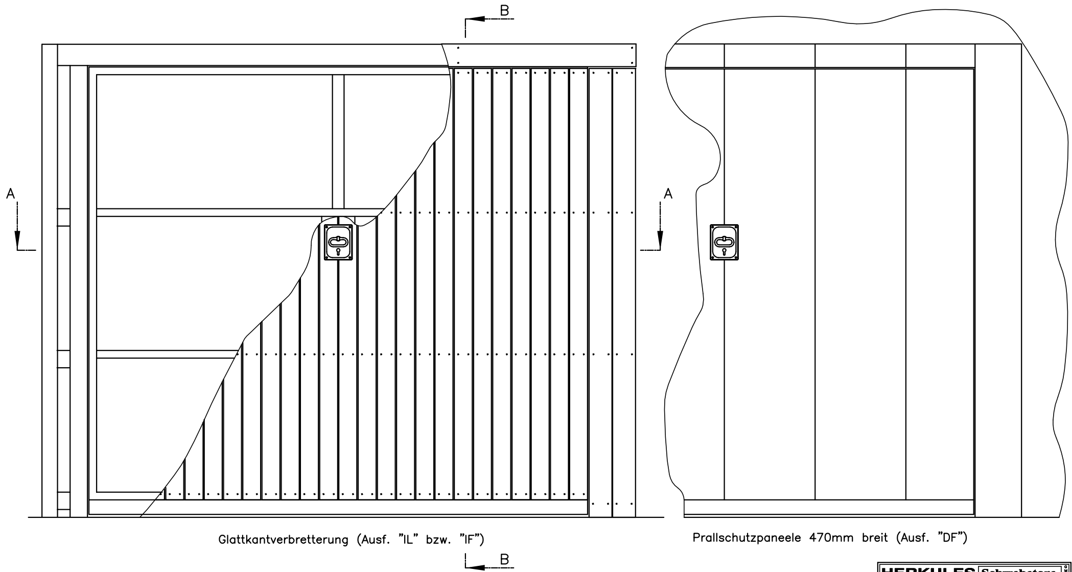
Ansicht Hallenseite
