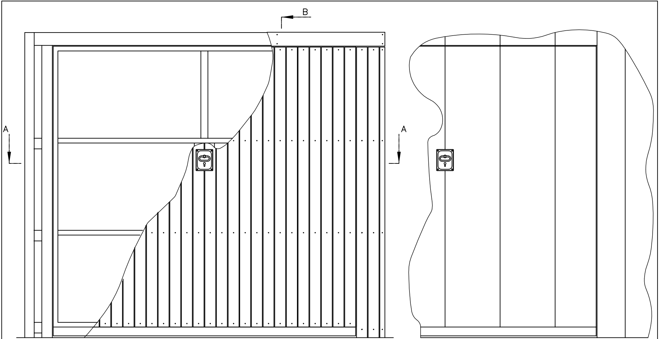
Profilholzverbretterung (Ausf. "I")
